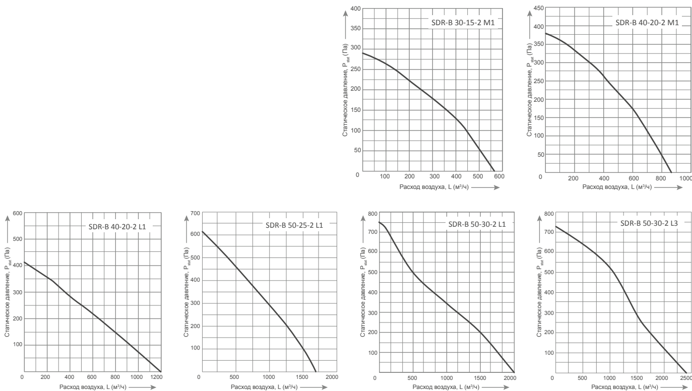
Схема 1 (230 В, 1 ф.)
