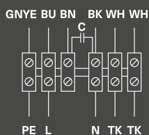
Схема 1 (230 В, 1 ф, 50 Гц.)
